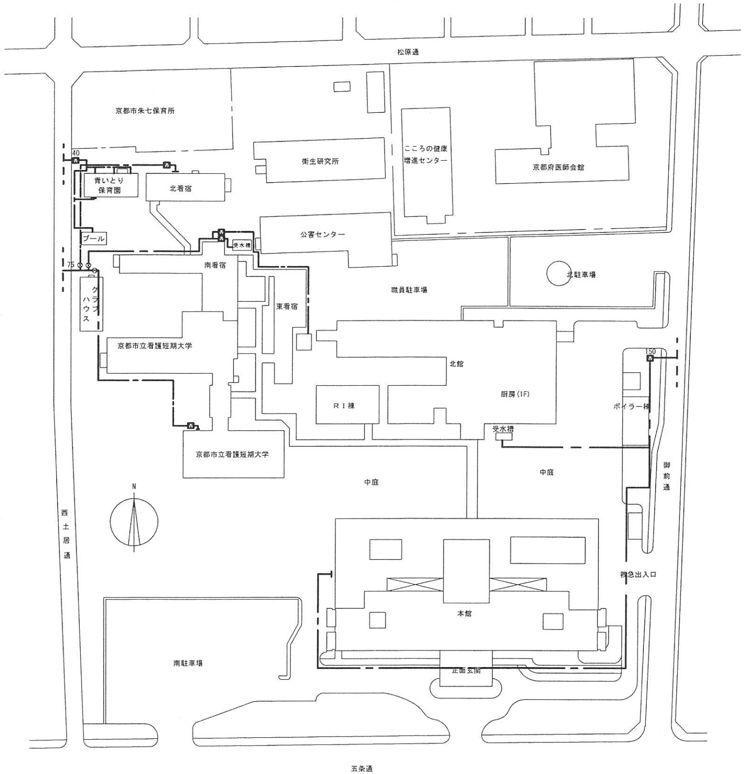
京都市立病院配置図（給水）
