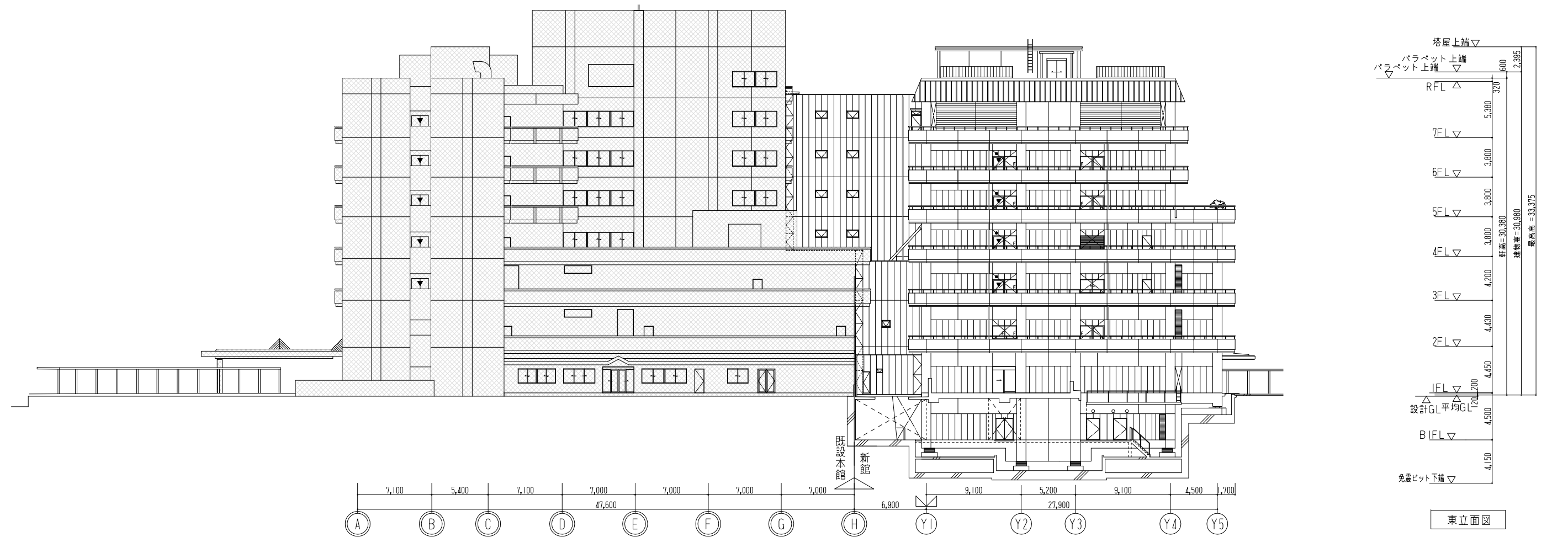
南立面図
