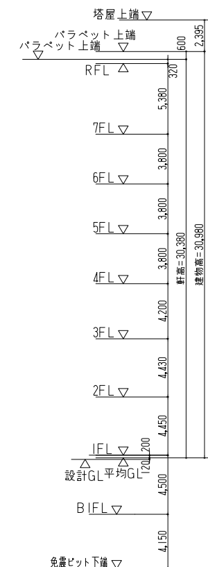
西立面図
