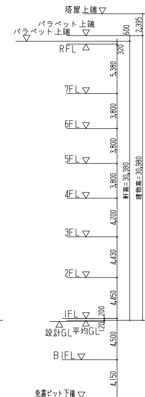
北立面図
