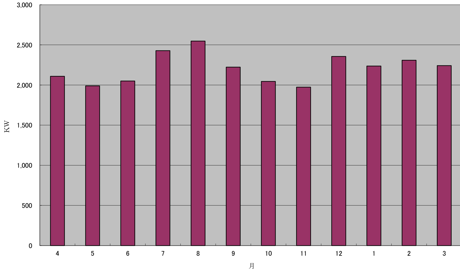
別表1参考図① 平成27年度 各月の最大需要電力
